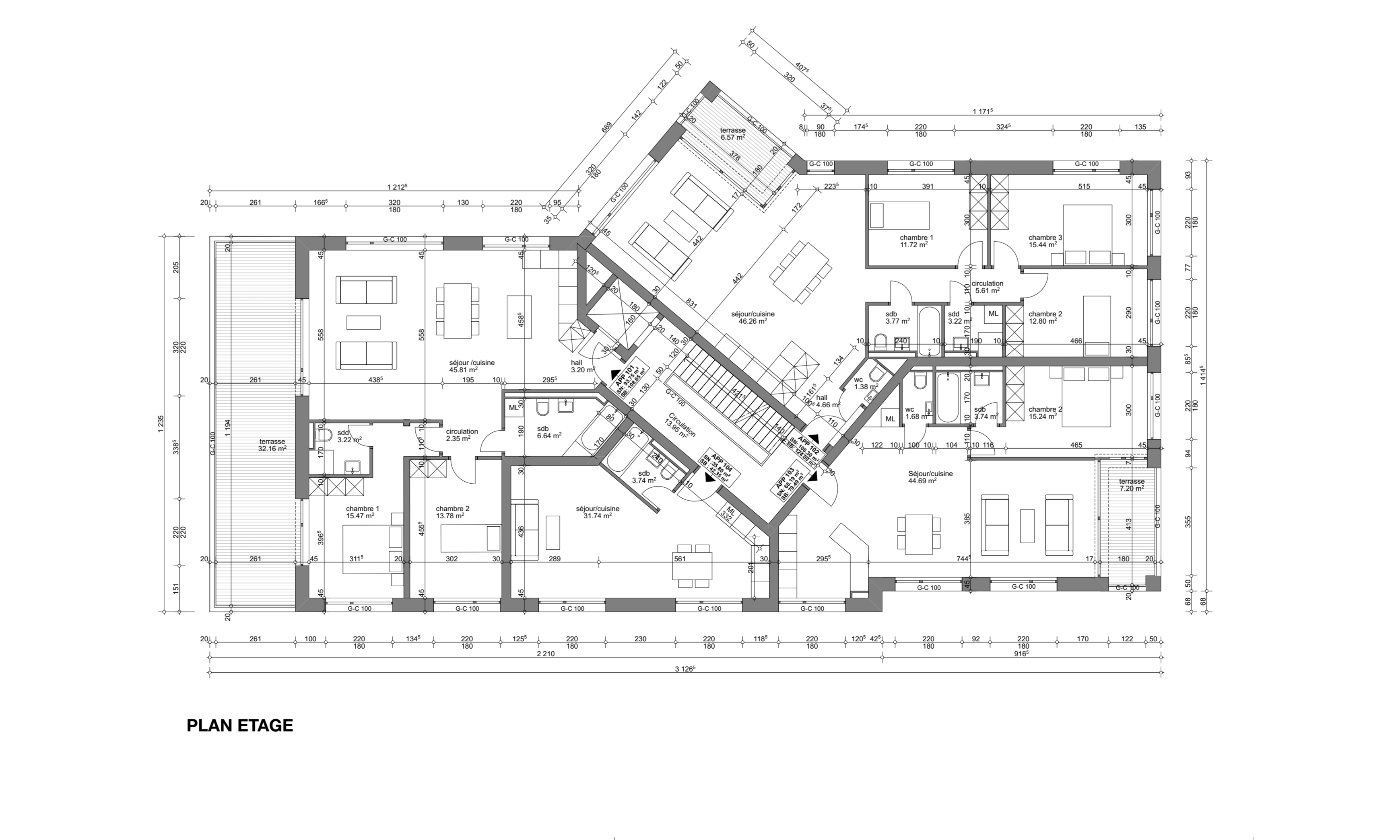
PLAN ETAGE
