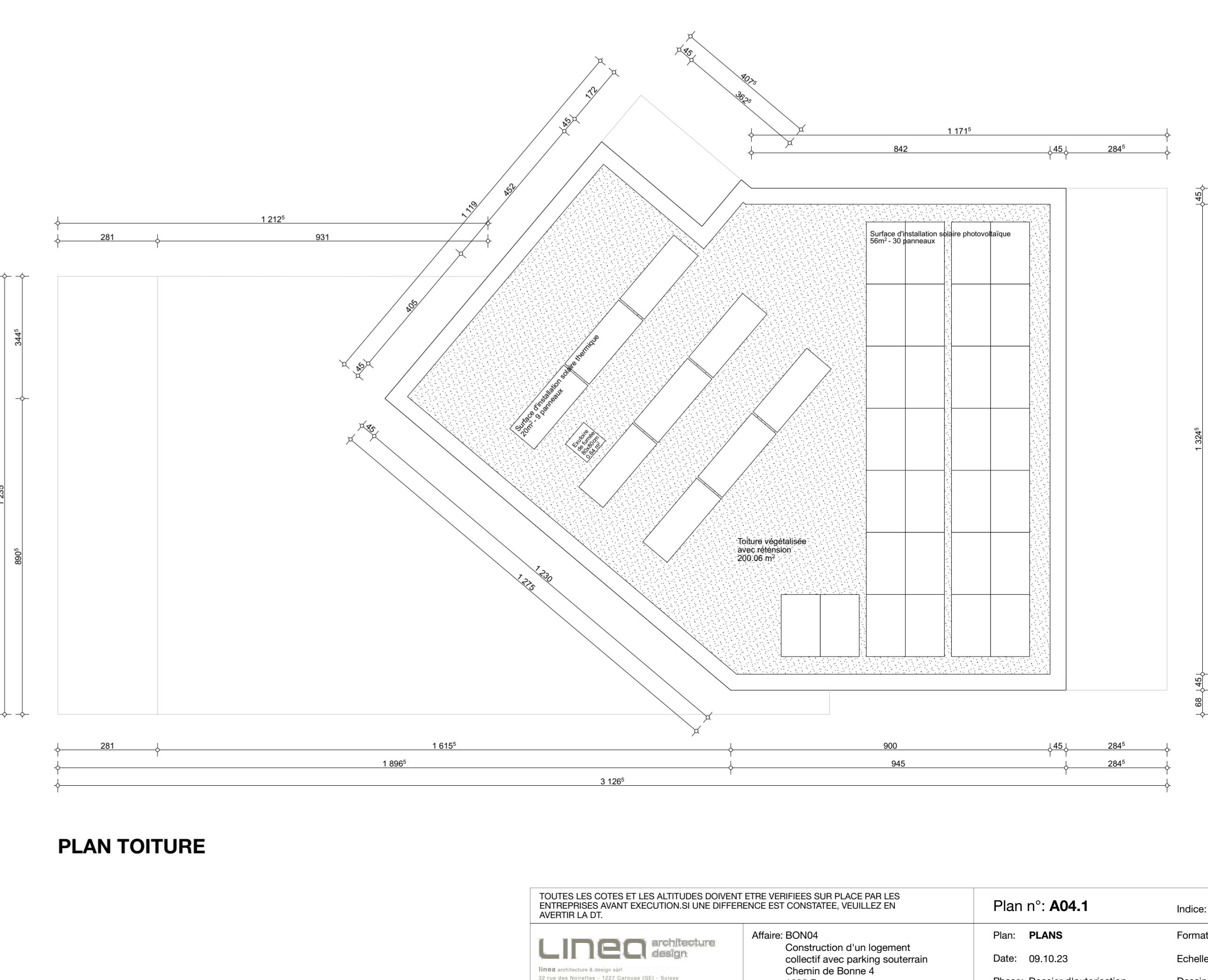
PLAN TOITURE
