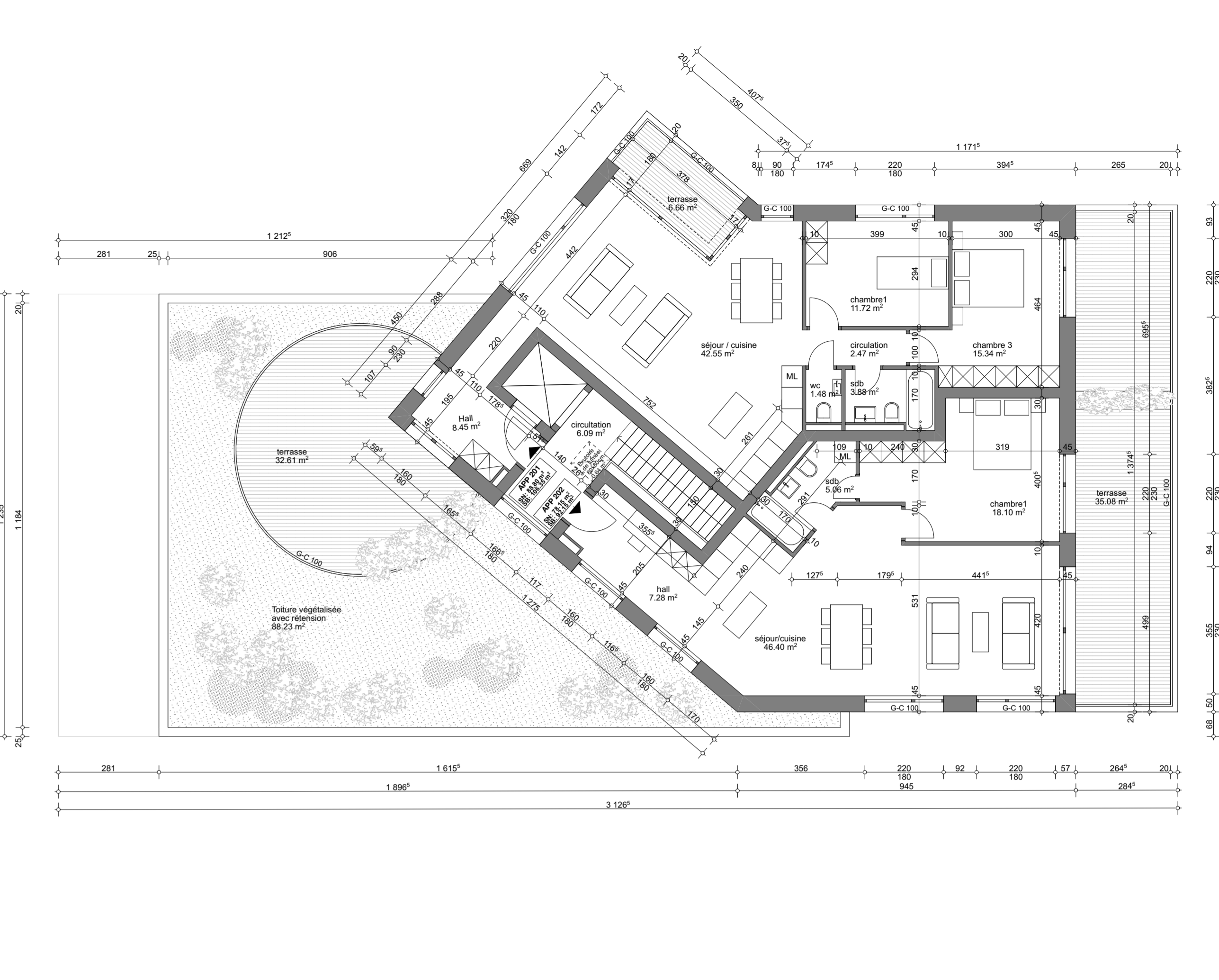
PLAN ATTIQUE
