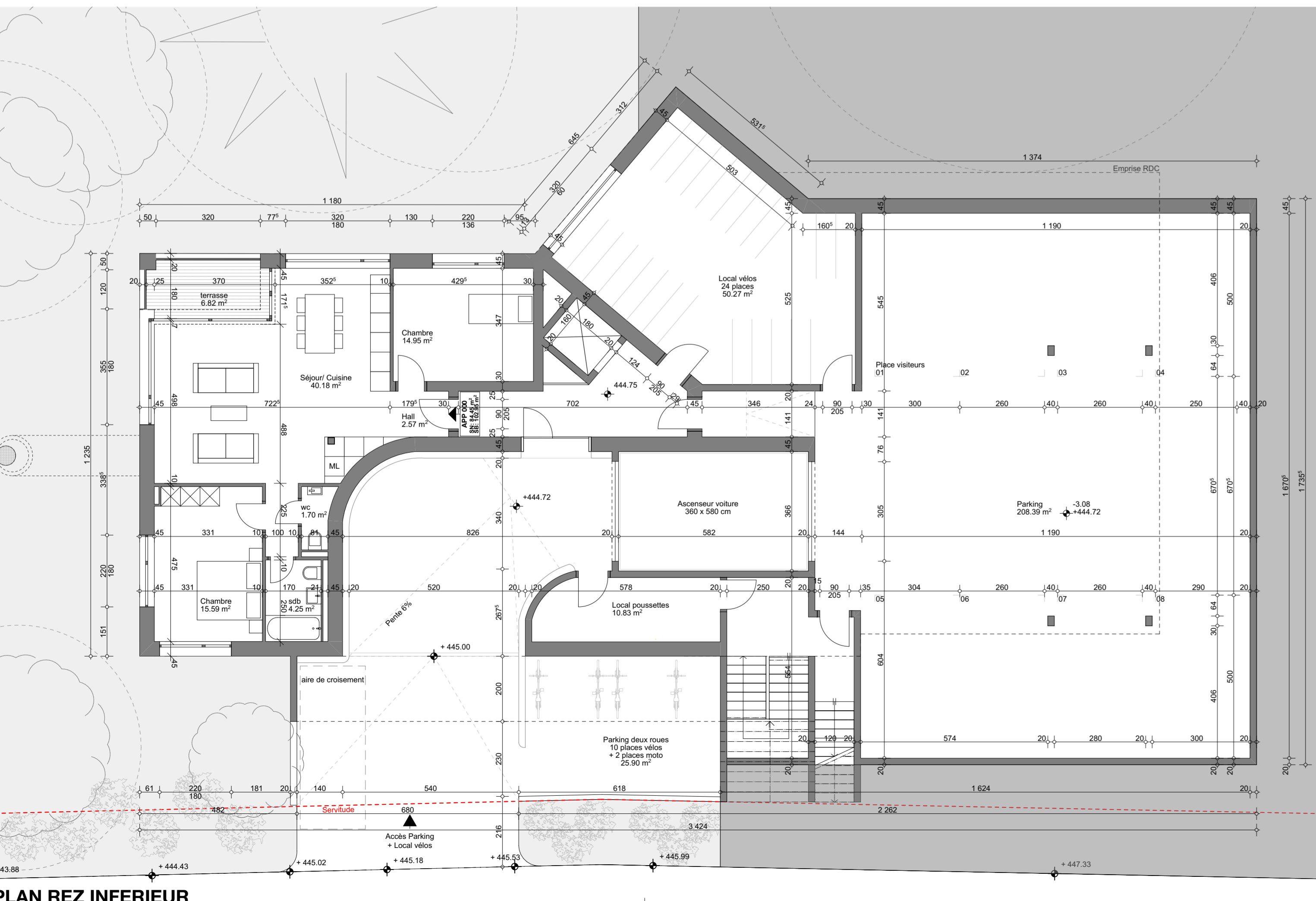
PLAN REZ INFÉRIEUR
