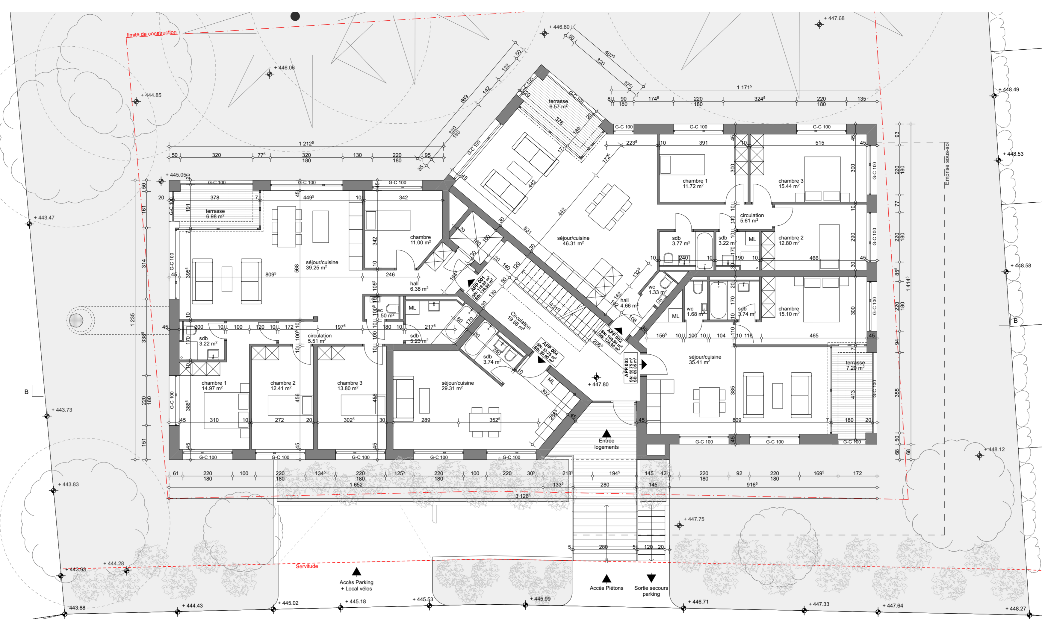
PLAN REZ SUPERIEUR
