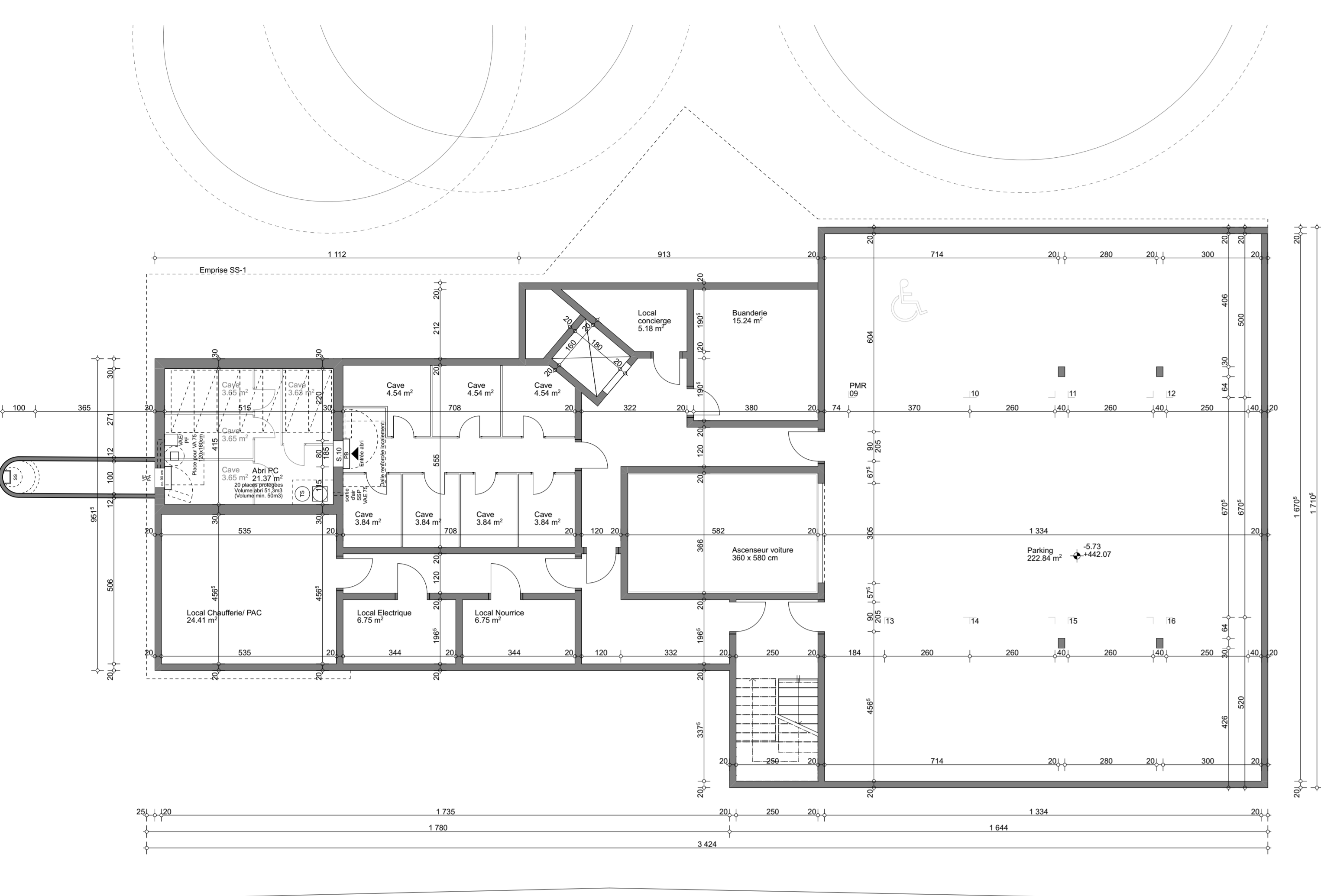
PLAN SOUS-SOL
